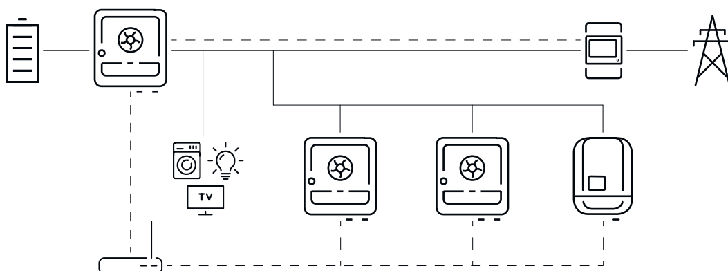
Exemplu schemă de conectare limitare dinamică a alimentării cu mai multe inverttoare
