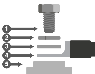
Conectarea cablului la baterie
