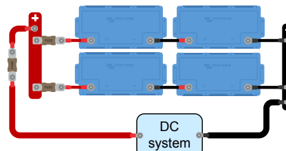
Mai multe baterii în serie/paralel
