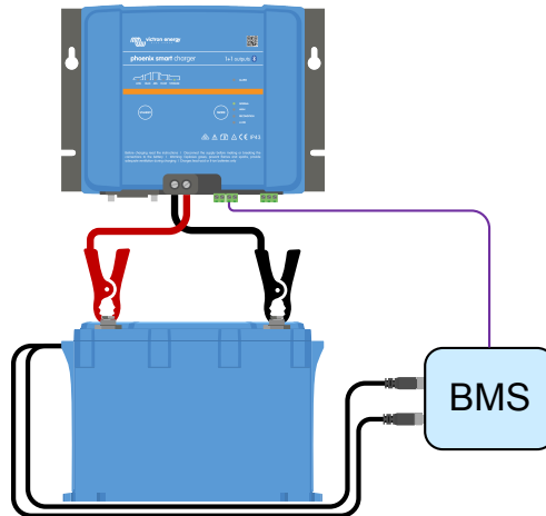
Încărcarea inițială folosind un BMS
