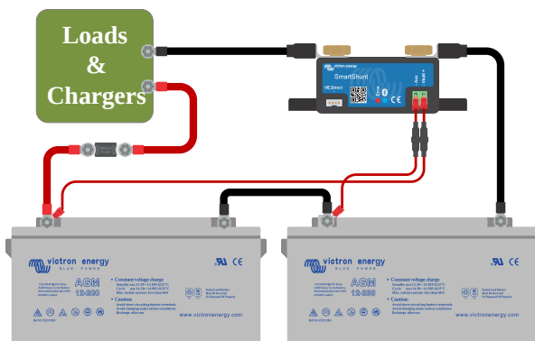
Sistem de monitorizare a bateriei cu sistem de monitorizare a punctului median auxiliar.
