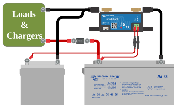
Sistem de monitorizare a bateriei cu sistem de monitorizare a bateriei suplimentare auxiliare.
