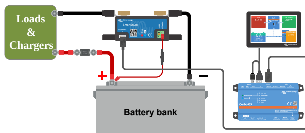
Sistemul de monitorizare a bateriei este conectat la un Cerbo GX și la un ecran GX Touch .
