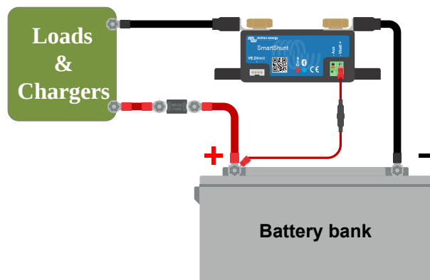
Instalarea sistemul de monitorizare a bateriei de bază.
