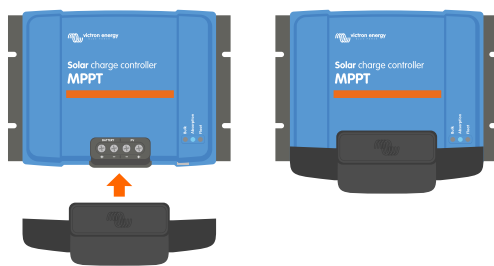
Exemplu încărcător solar cu MPPT WireBox
